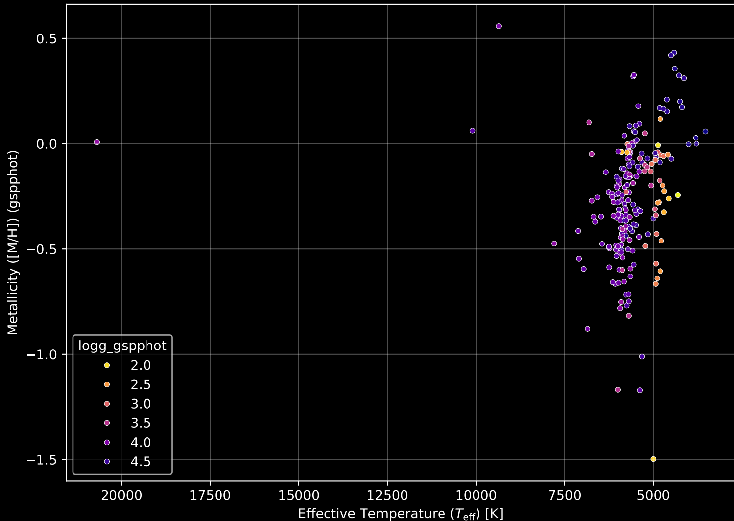
APOGEE DR17 Field: [K2_C3_043-50] Stellar Population Parameters (n= 208)
